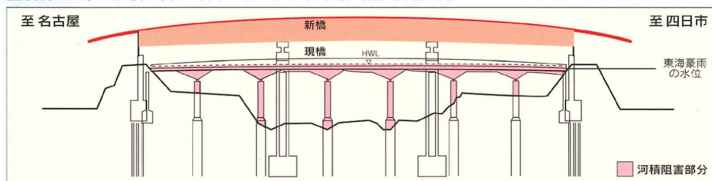
■橋脚は2本に、橋の高さも嵩上げされます (現橋と新橋の横断模式図)
