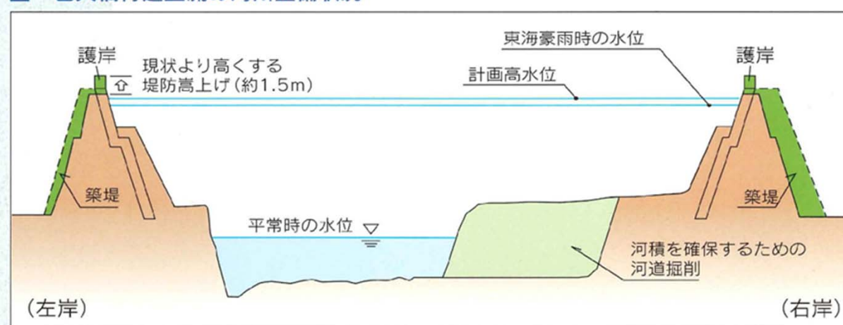
■一色大橋付近上流の河川整備状況
