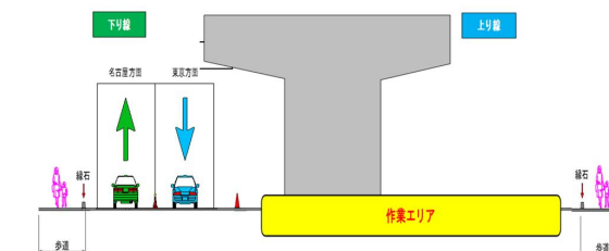
下り線対面通行イメージ
