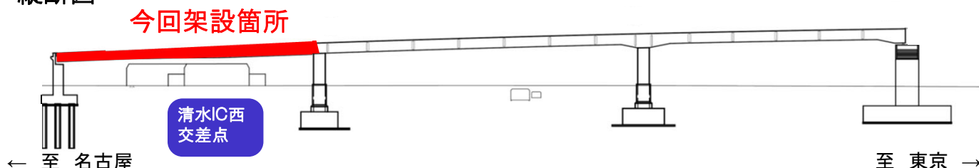
縦断面図
