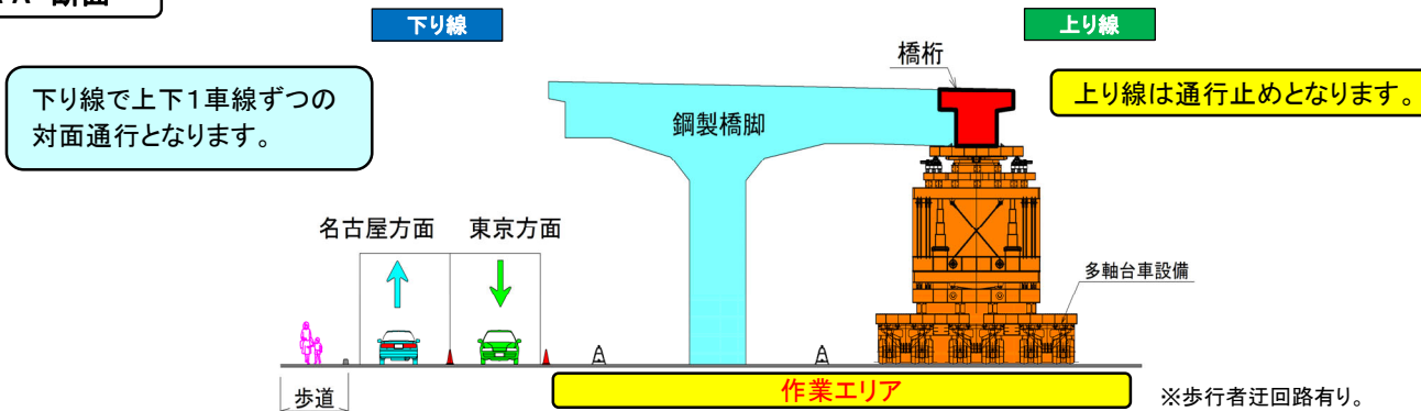
A-A 断面
