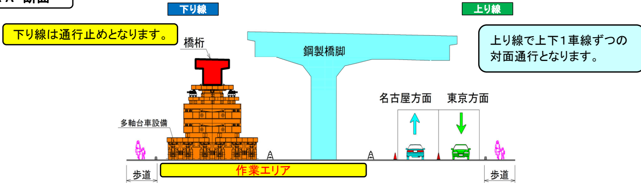
A-A 断面
