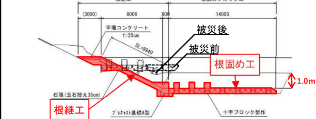
【断面図】
