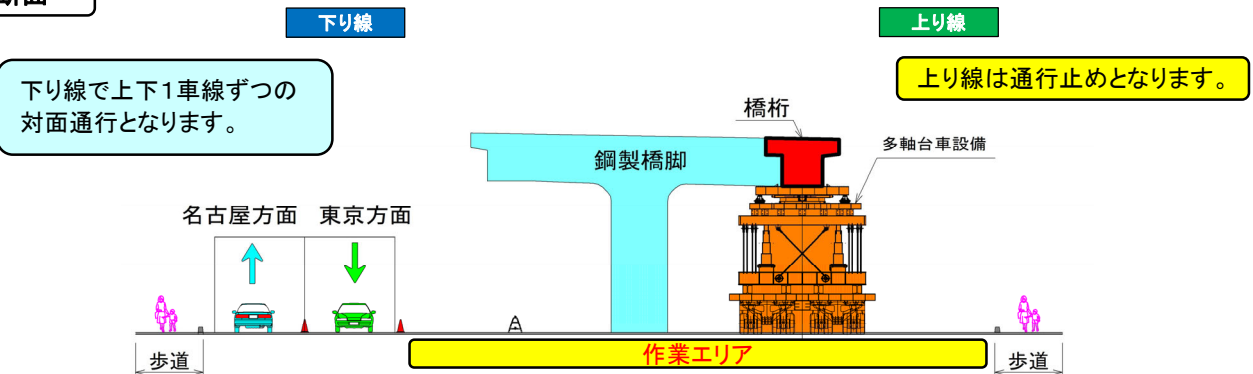
A-A 断面
