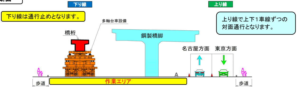
A-A 断面
