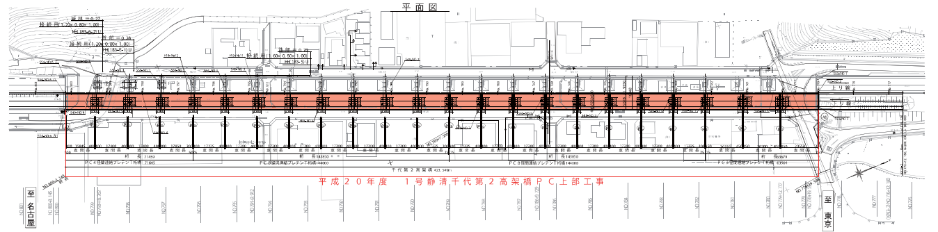
平面図
