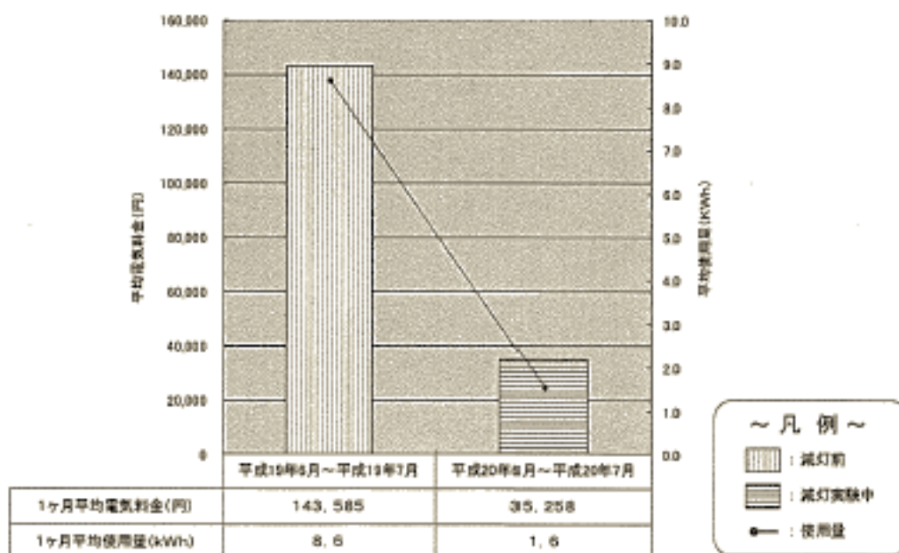
減灯実験前後の電気使用量および電気料金の推移グラフ (対前年比)
