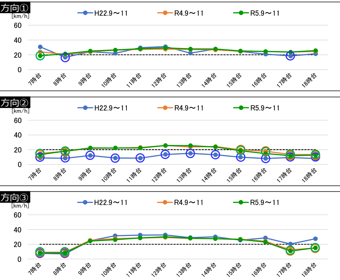
出典：民間プローブデータ（H22.9～11月平日）、ETC2.0プローブデータ（R4・5.9～11月平日）により算出
