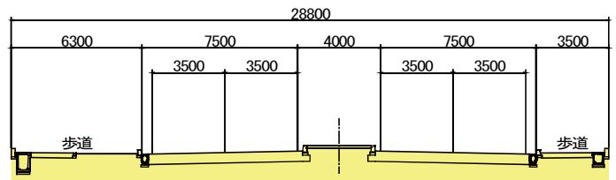
東海道新幹線交差部 C-C 断面
