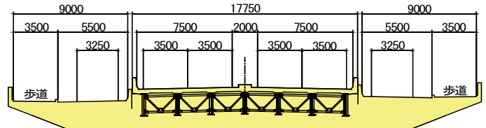
JR 東海道線交差部 A-A 断面
