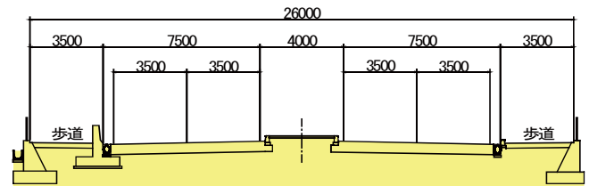
土工部 B-B 断面
