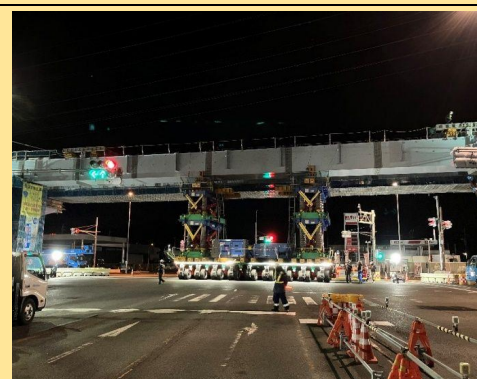
庵原高架橋鋼上部工事 工事進捗状況
