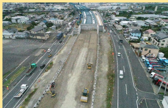
尾羽地区道路建設工事 工事進捗状況
