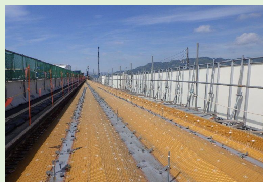
飯田地区南道路建設工事 工事進捗状況
