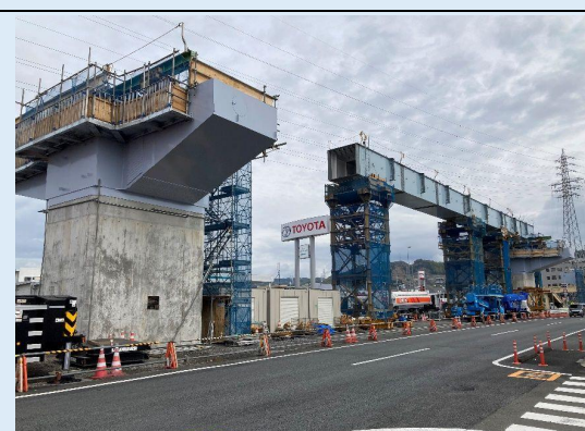
庵原高架橋鋼上部工事 工事進捗状況
