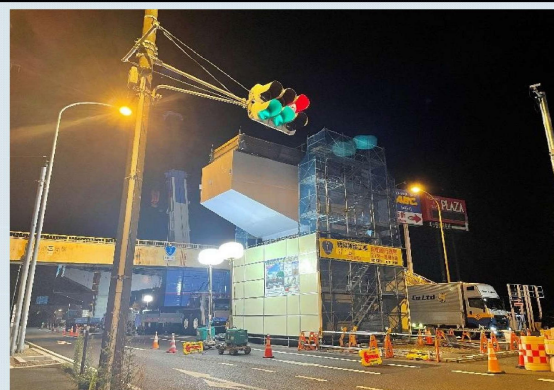
庵原高架橋東鋼製梁工事
