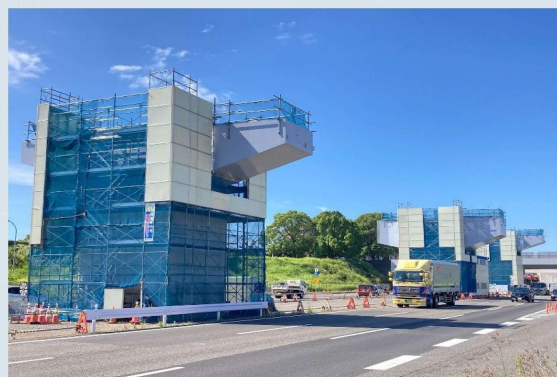
清水IC第2高架橋鋼製梁 工事進捗状況
