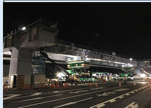
八坂高架橋 P31～P32主桁架設状況
