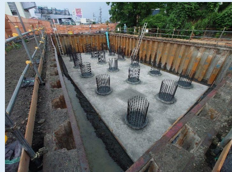
清水IC Fランプ橋台・擁壁底板部施工状況
