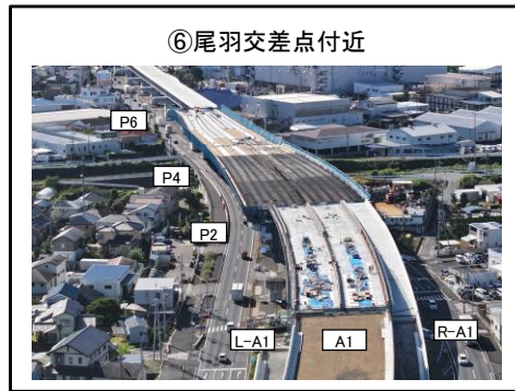
P2橋脚～P6橋脚 床版工 施工中 A1橋台～P2橋脚 床版工 施工中
