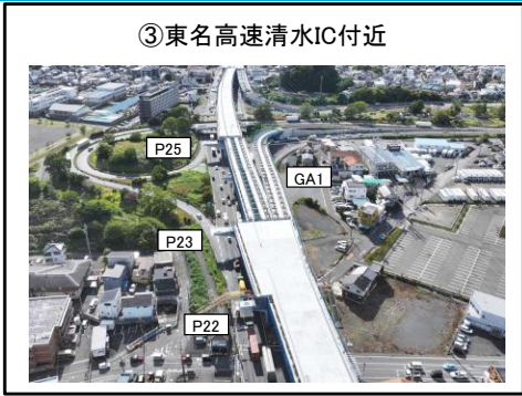
GA1～P23橋脚 床版工 施工中 P23～P25橋脚 上部工 施工中
