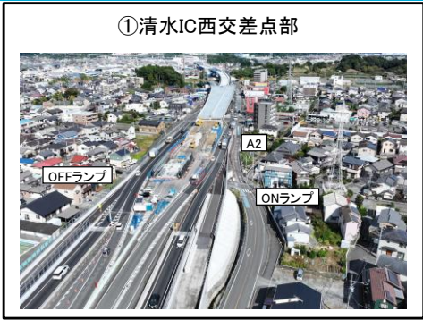
A2橋台西側擁壁部 擁壁工 施工中
