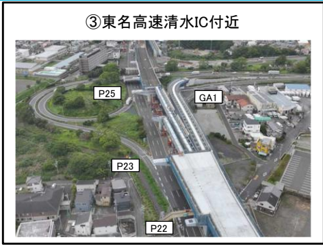
P19〜P23橋脚 床版工 施工中 P23〜P25橋脚 上部工 施工中
