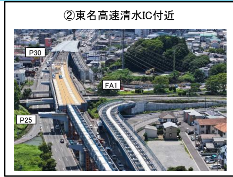
FA1~P30橋脚 上部工 施工中 P25~P30橋脚 床版工 施工中
