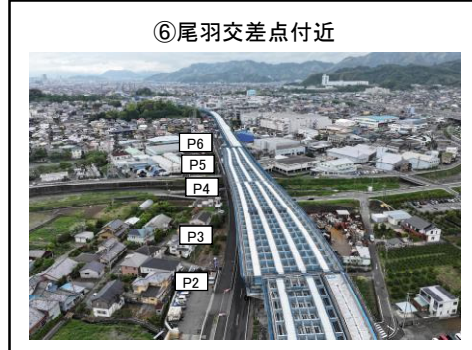
P2橋脚～P6橋脚 床版工 施工中
