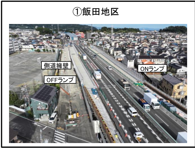
飯田ON・OFFランプ合流部 床版工 施工中 側道 擁壁 施工中
