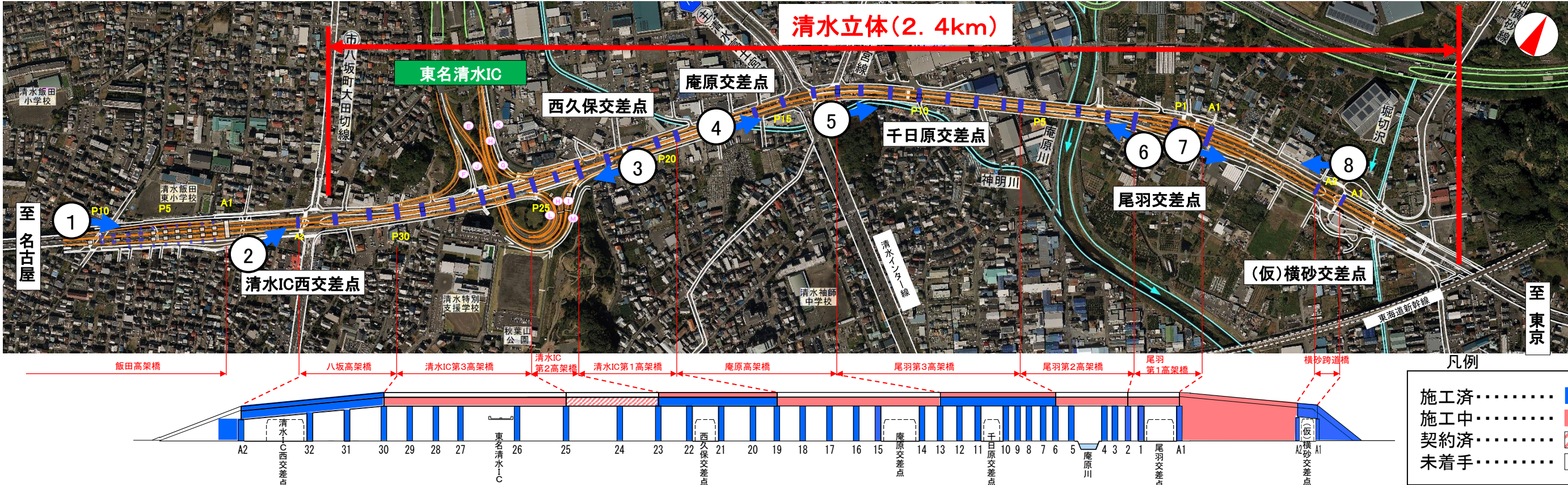
GP2橋脚 下部工 施工完了 P19～P23橋脚 床版工 施工中 P25～P30橋脚 上部工 施工中
