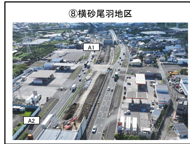
A1橋台、A2橋台間 擁壁工 施工中
