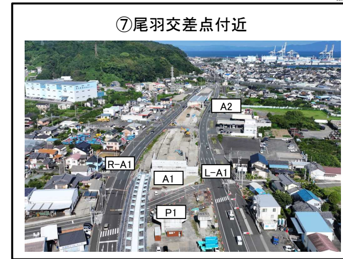
A1橋台、A2橋台間 擁壁工 施工中 A1橋台~P2橋脚 上部工 準備中 A1橋台~P2橋脚 オフランプ床版工 施工中
