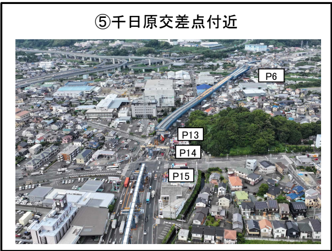
P6橋脚～P13橋脚 床版工 施工中
