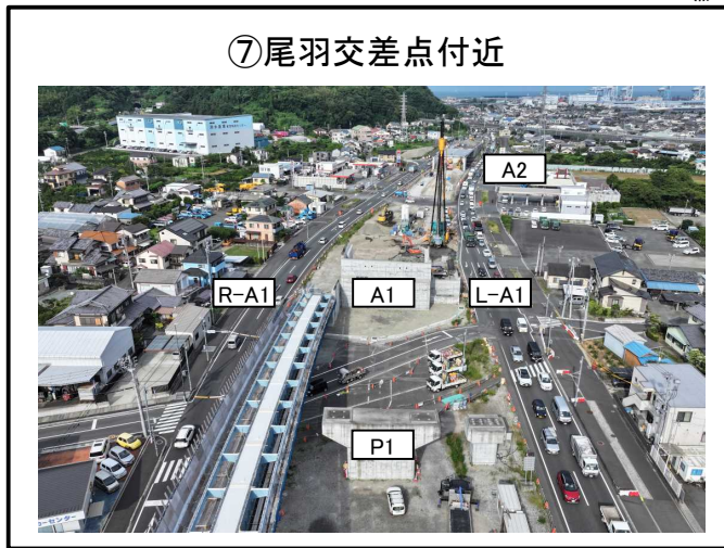
A1橋台、A2橋台間 擁壁工 施工中 A1橋台～P2橋脚 上部工 準備中 A1橋台～P2橋脚 オフランプ 施工中
