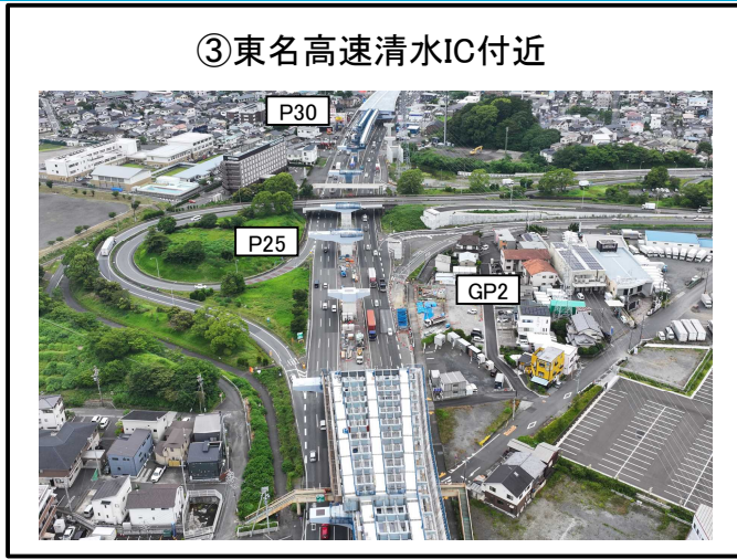
GP2橋脚 下部工 施工中 P25～P30橋脚 上部工 施工中
