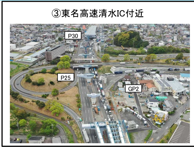
③東名高速清水IC付近 GP2橋脚 下部工 施工中 P25～P30橋脚 上部工 施工中
