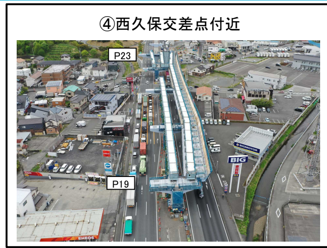
④西久保交差点付近 P19～P23橋脚 上部工 施工中
