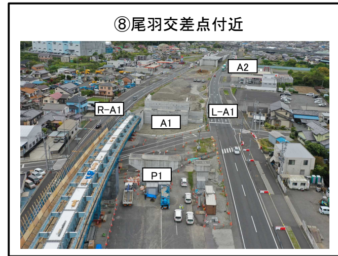
⑧尾羽交差点付近 A1橋台、A2橋台間 擁壁工 準備中 A1橋台～P2橋脚 上部工 準備中 A1橋台～P2橋脚 オフランプ 施工中
