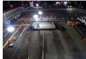
P22橋脚覆工板設置状況
