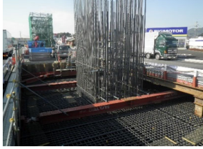
P19 橋脚施工状況
