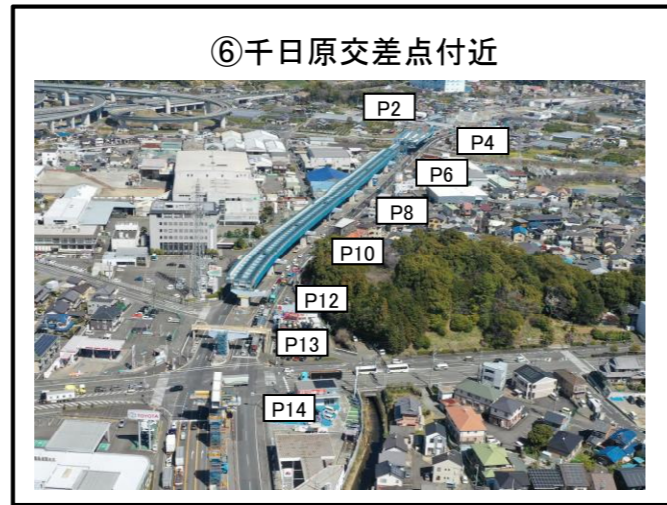
⑥千日原交差点付近 P6橋脚~P13橋脚 上部工 施工完了
