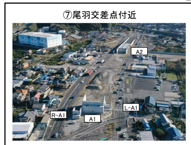
⑦尾羽交差点付近 A1橋台、A2橋台間 地盤改良 施工中
