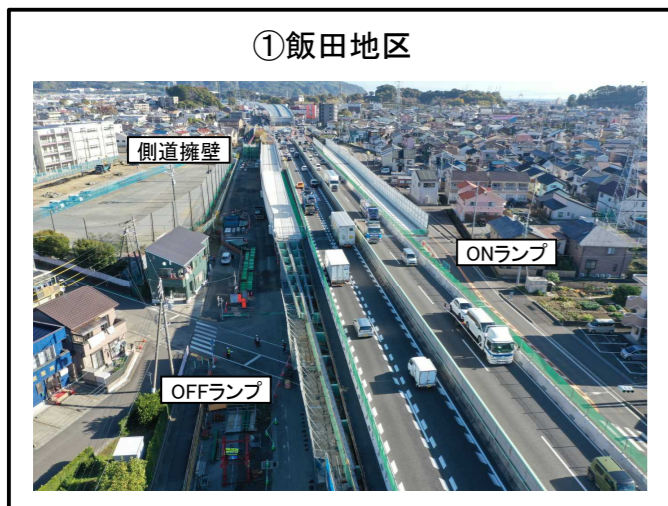
①飯田地区 飯田ON・OFFランプ合流部 上部工 施工中 側道 擁壁 施工中
