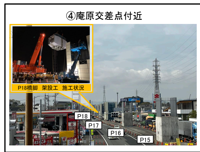
P18橋脚 鋼製梁架設 施工中
