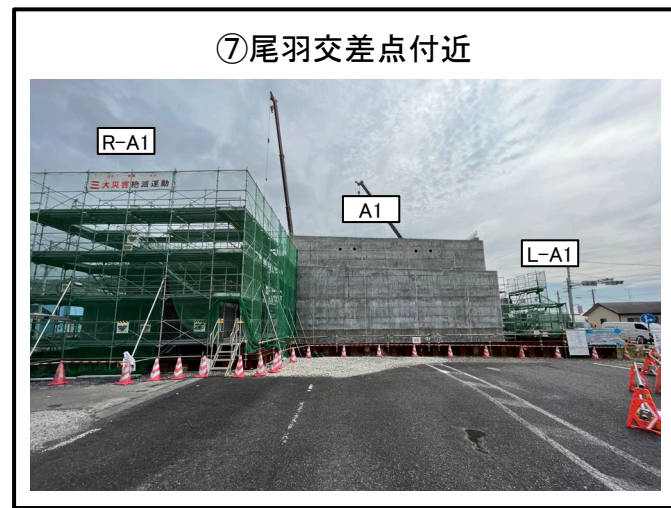
R-A1橋台、L-A1橋台 下部工 施工中
