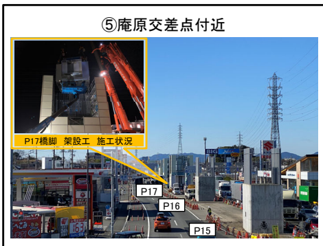
P17橋脚 鋼製梁架設 施工中
