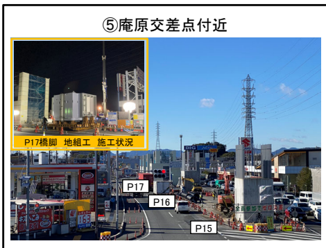
P17橋脚 鋼製梁架設 準備中
