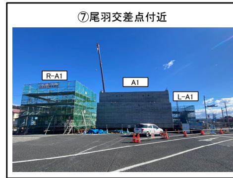
R-A1橋台、L-A1橋台 施工中
