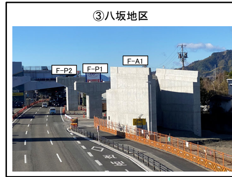
清水IC F-A1~F-P2橋脚 下部工 施工完了
