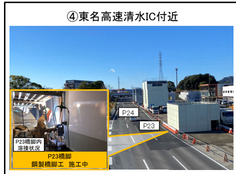
P23橋脚 鋼製橋脚工 施工中
