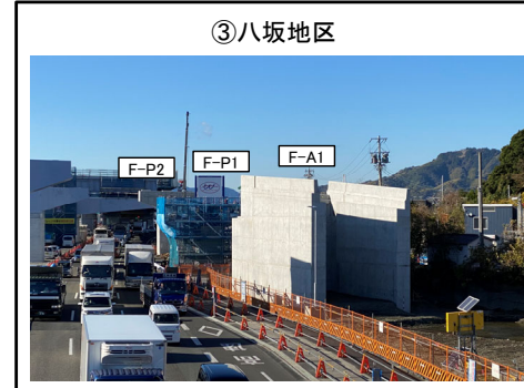
清水IC F-P1橋脚 下部工 施工中
