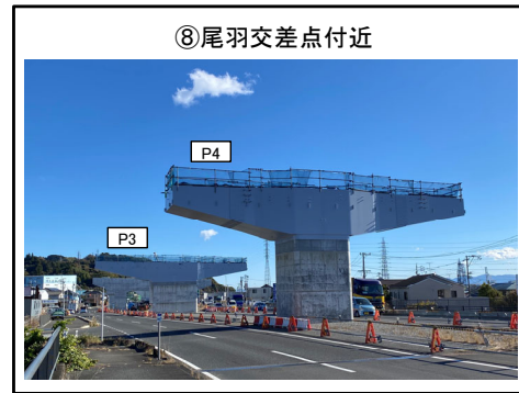
P3~P4橋脚 鋼製梁 施工完了
