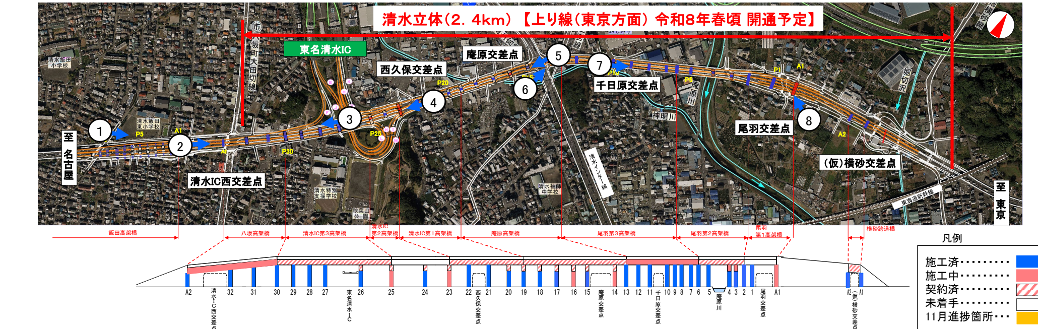
飯田OFFランプ橋 上部工 施工中
