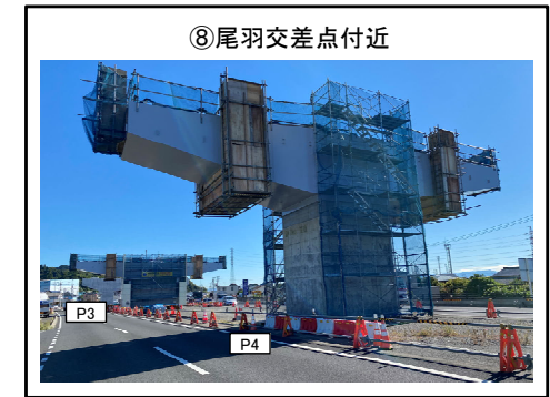
P3橋脚～P4橋脚 鋼製梁 張出部架設完了
