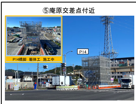
P14橋脚 躯体工 施工中
