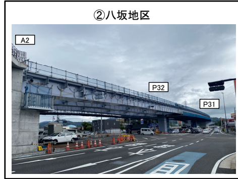
A2橋台～P30橋脚 主桁 架設完了
