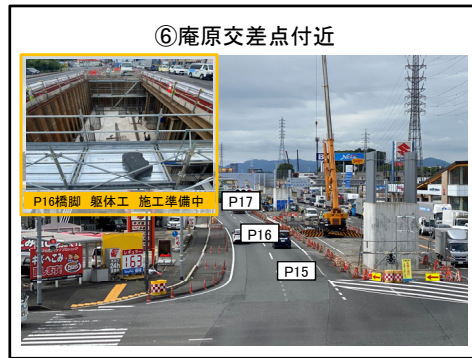
P16橋脚 躯体工 施工準備中
