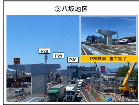
P29橋脚 鋼製梁工 施工完了
