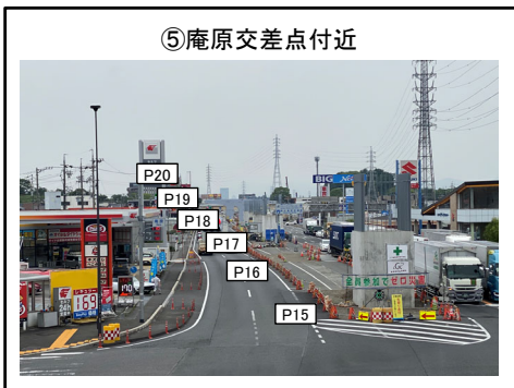
P16橋脚 仮設工 施工中
