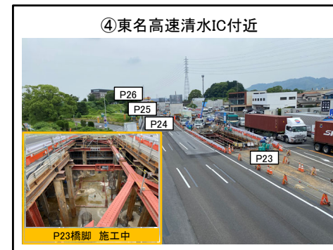
P23橋脚 P25橋脚 施工中
