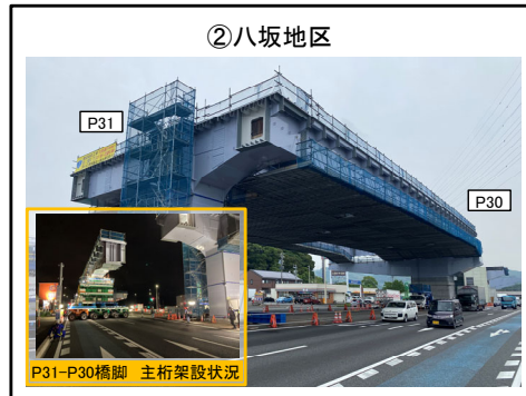
P31橋脚~P30橋脚 主桁架設(4本/4本)完了
