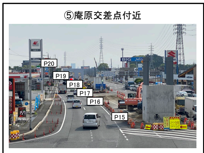
P16橋脚 仮設工 施工中
