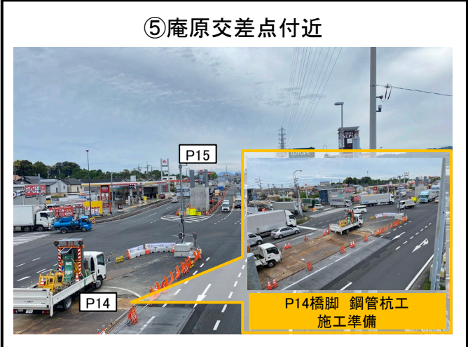
⑤庵原交差点付近 P14橋脚 鋼管杭工 施工準備
