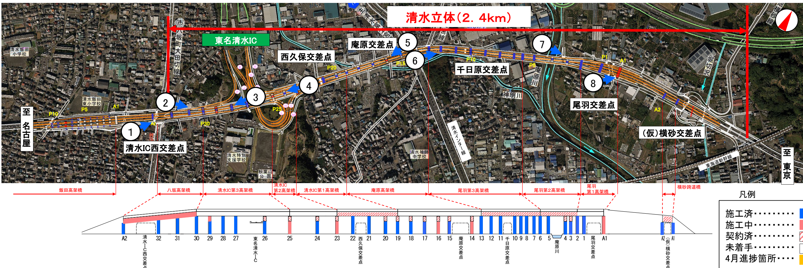
①清水IC西交差点付近 A2橋台～P32橋脚 主桁架設(1本/3本)完了
