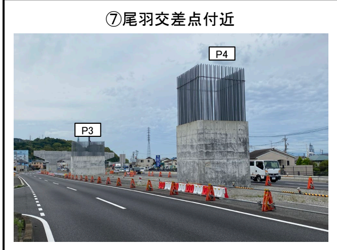
⑦尾羽交差点付近 P3橋脚 P4橋脚 鋼製梁工 施工準備
