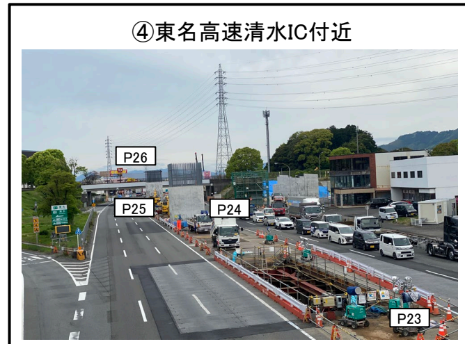
④東名高速清水IC付近 P23橋脚 P25橋脚 施工中
