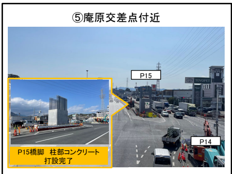
P15橋脚 柱部コンクリート打設 完了
