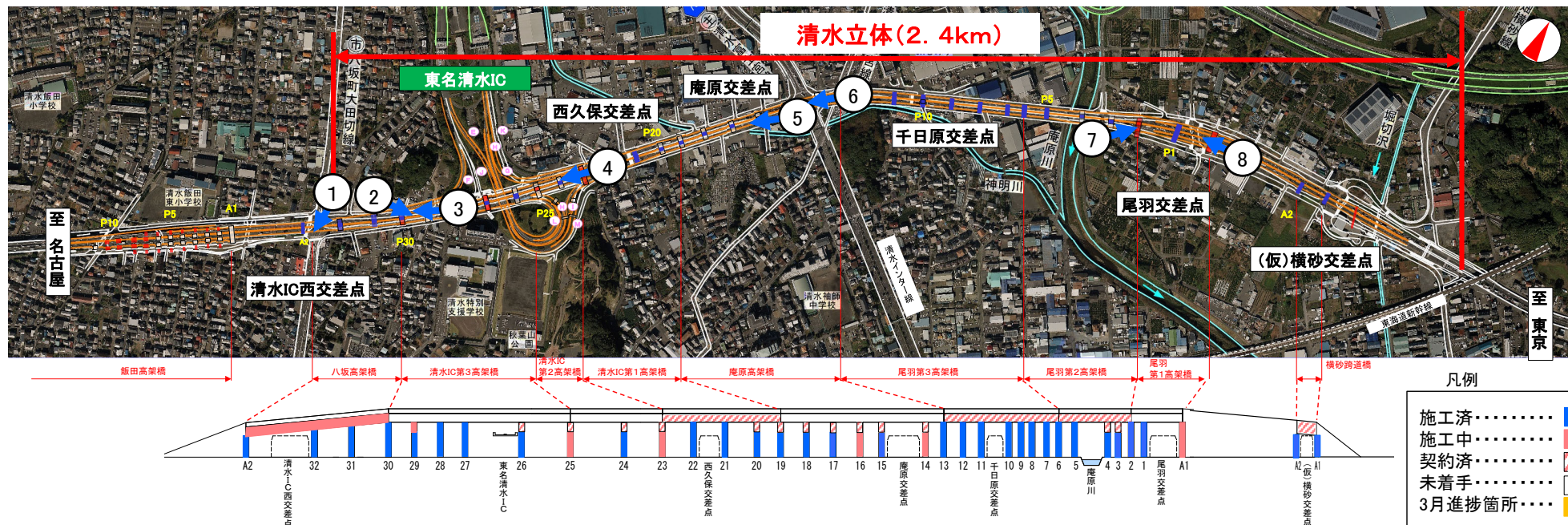
A2橋台～P32橋脚 主桁架設(1本/3本)完了
