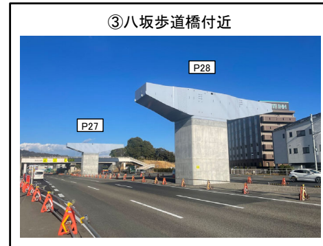
P27橋脚、P28橋脚 工事完成
