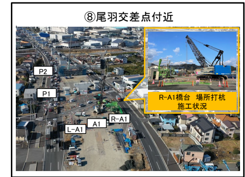
R-A1橋台 場所打杭に着手
