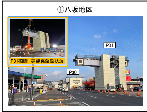
P30橋脚、P31橋脚 鋼製梁の架設完了
