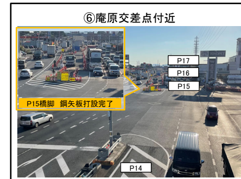
⑥庵原交差点付近 P15橋脚 鋼矢板打設完了
