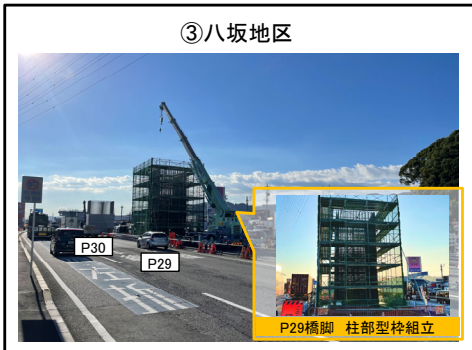
③八坂地区 P29橋脚 柱部型枠組立に着手
