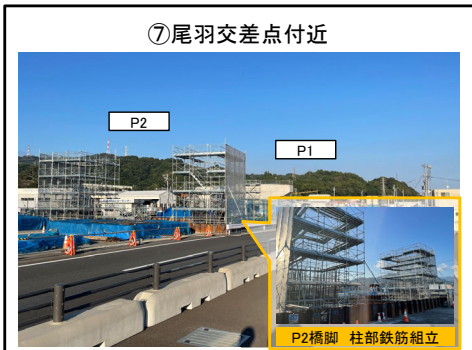
⑦尾羽交差点付近 P2橋脚 柱部鉄筋組立に着手
