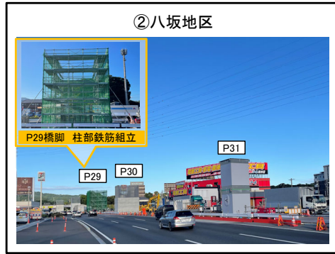
P29橋脚 柱部鉄筋組立に着手
