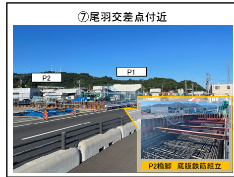
P2橋脚 底版鉄筋組立に着手
