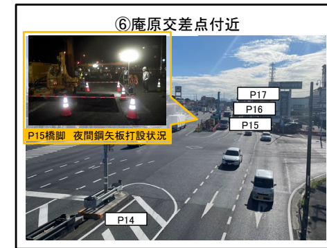
P15橋脚 鋼矢板打設に着手
