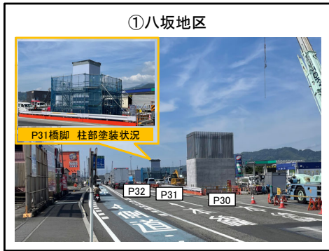
①八坂地区 P31橋脚 鋼製柱の塗装工に着手
