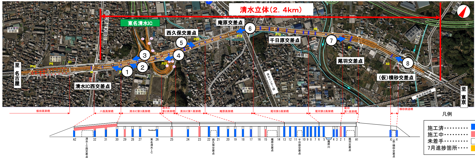
①八坂地区 P31橋脚 鋼製柱の塗装工に着手
