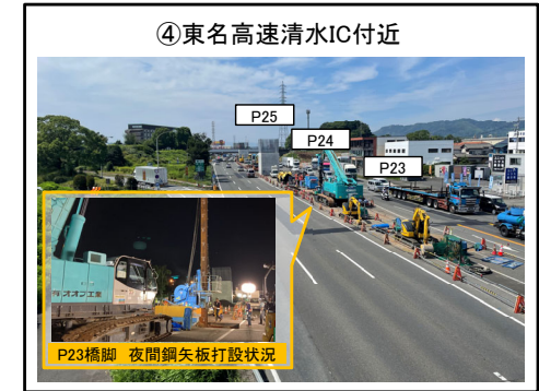
④東名高速清水IC付近 P23橋脚 鋼矢板打設に着手
