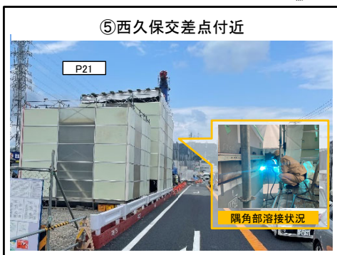
P21橋脚 隅角部の溶接に着手
