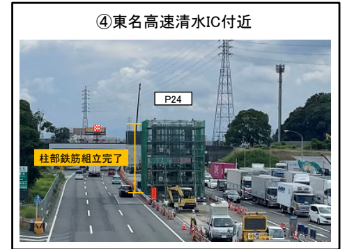
P24橋脚 柱部の鉄筋組立完了
