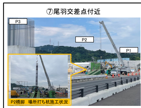
P2橋脚 場所打ち杭に着手(13/20本完了)
