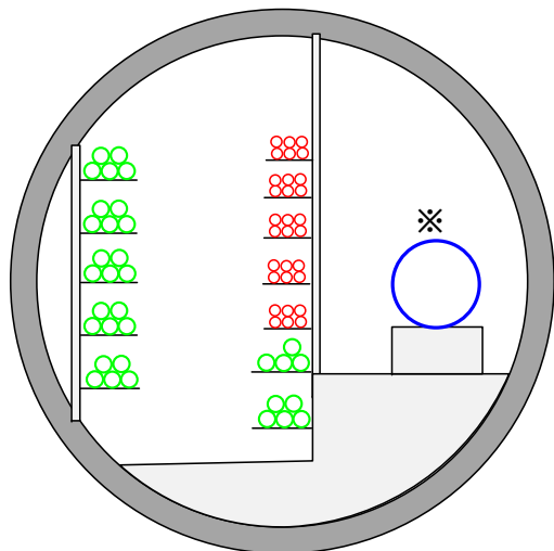
標準断面図（シールド区間（清水地区））
