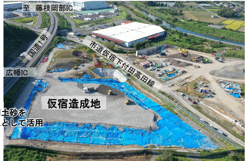
② 仮宿造成地の状況
